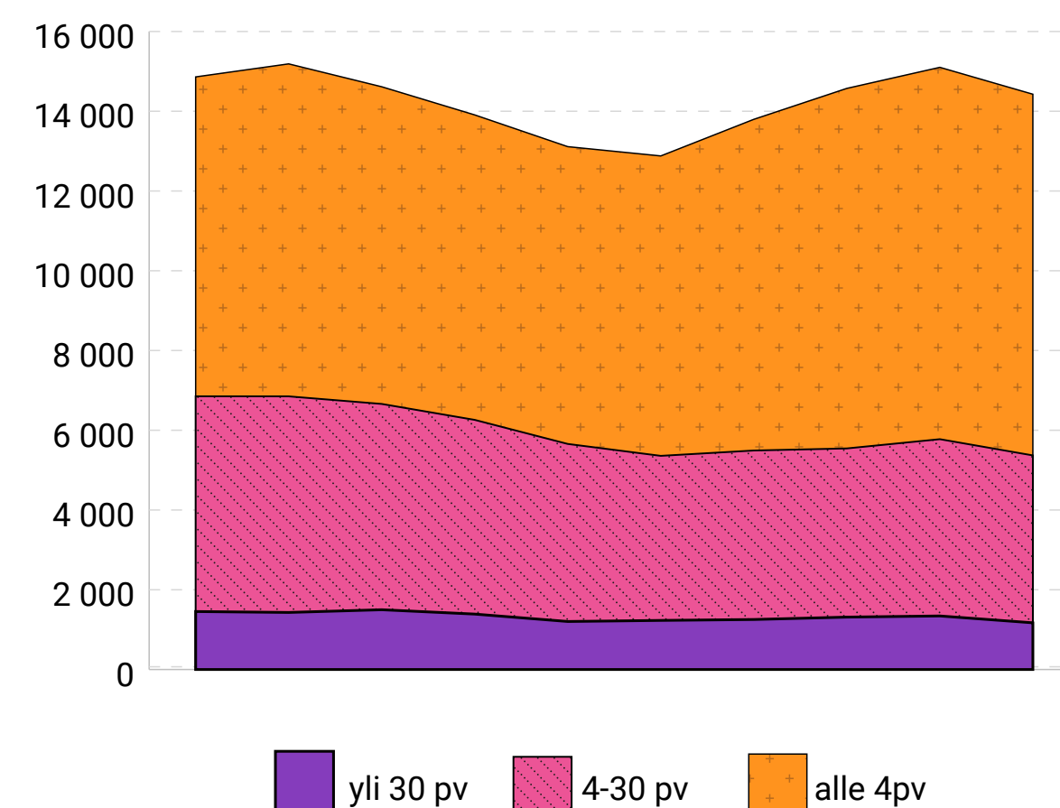
Kuvaaja 3. Rakennustyömailla sattuneet työpaikkatapaturmat vuosina 2016-2019
